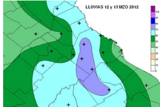
Figura 10: Lluvias 12 y 13 de marzo de 2012
