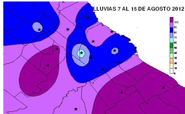
Figura 18: Lluvias (mm) 7-8, 11-12 y 14-15/8/2012.
