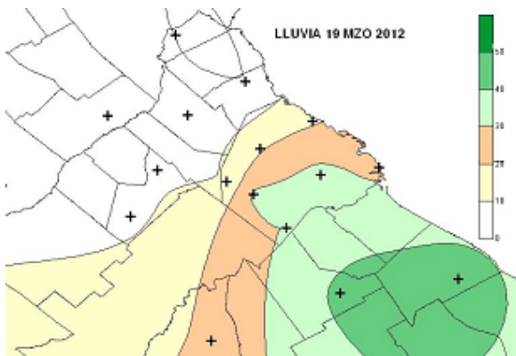
Figura 11: Lluvias 19 de marzo de 2012
