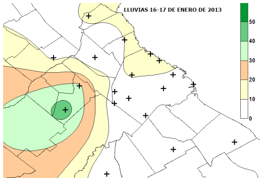
Figura 33: Lluvias (mm) 16-17 de enero de 2013
