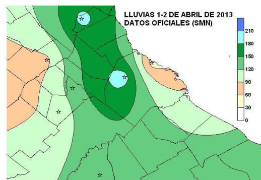
Figura 36: Lluvias del 1-2 de abril de 2013
