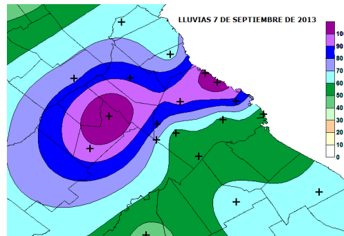
Figura 40: Lluvias 7 de septiembre de 2013
