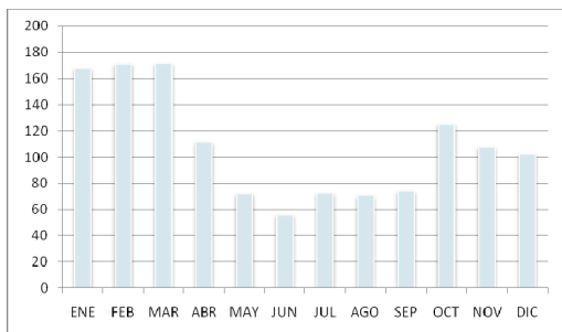
Figura 3: Precipitación media mensual en el OCBA (2001/10).
