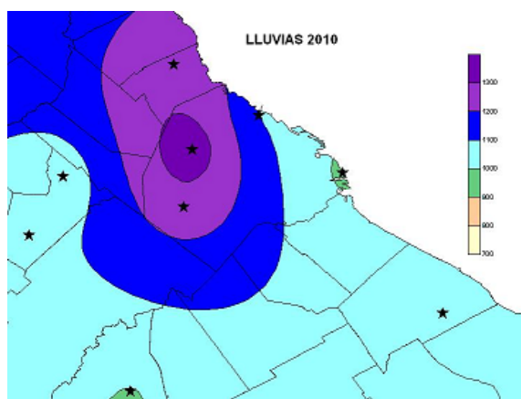
Figura 31: Lluvias totales (mm) en 2010
