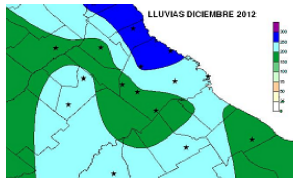
Figura 28: Lluvias totales (mm) en diciembre.
