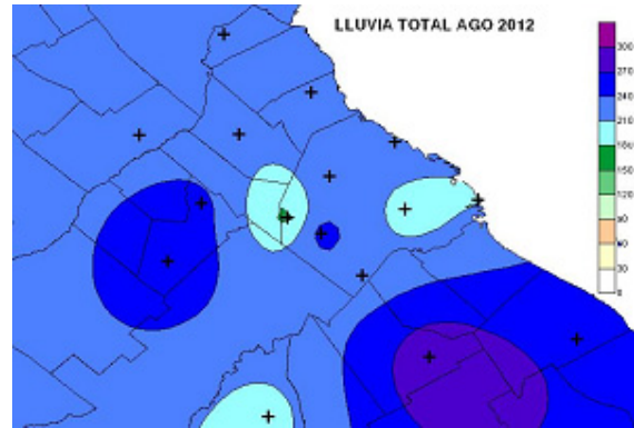
Figura 20: Lluvias totales (mm) agosto de 2012.
