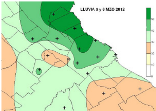
Figura 9: Lluvias 5 y 6 de marzo de 2012
