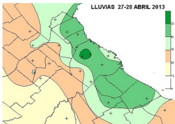
Figura 37: Lluvias 27-28 de abril de 2013
