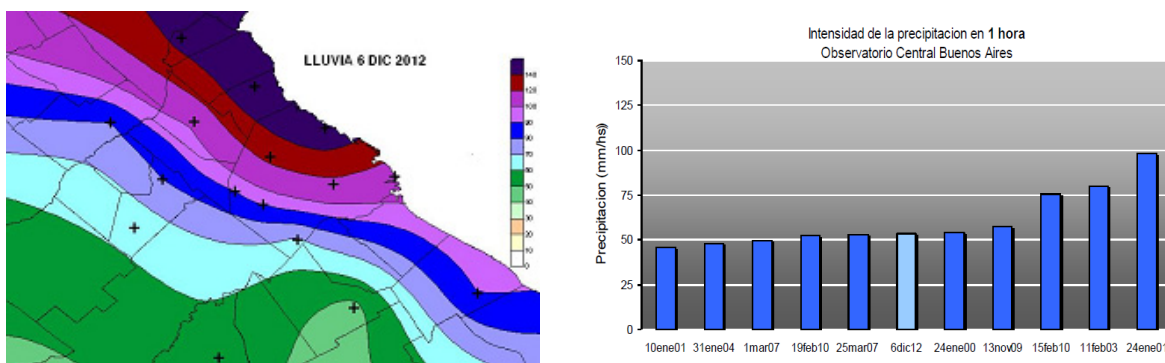
Figura 25: Lluvias (mm) 6 de diciembre de 2012
