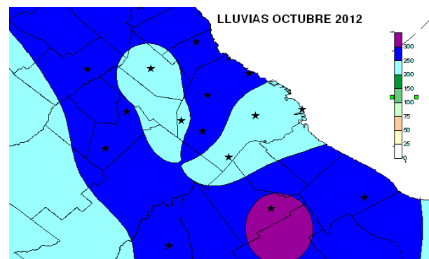
Figura 22: Lluvias totales (mm) octubre de 2012.
