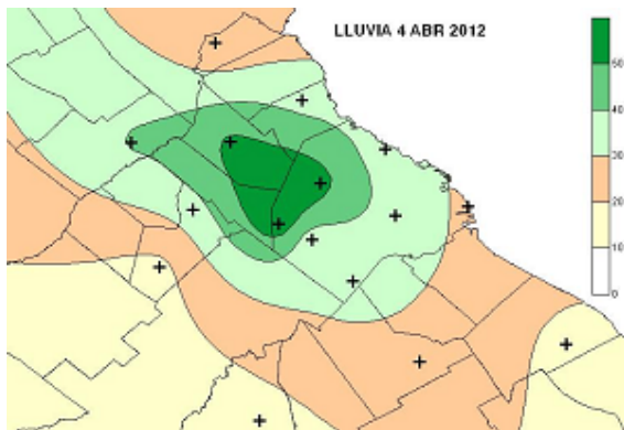
Figura 13: Lluvias (mm) 4 de abril de 2012
