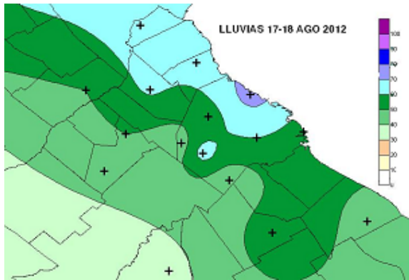
Figura 19: Lluvias (mm) 17-18 de agosto de 2012
