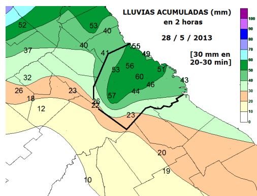
Figura 38: Lluvias del 28 de mayo de 2013
