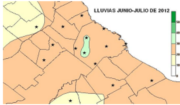
Figura 15: Lluvias (mm) marzo-abril-mayo de 2012 Figura 16: Lluvias (mm) junio-julio de 2012.
