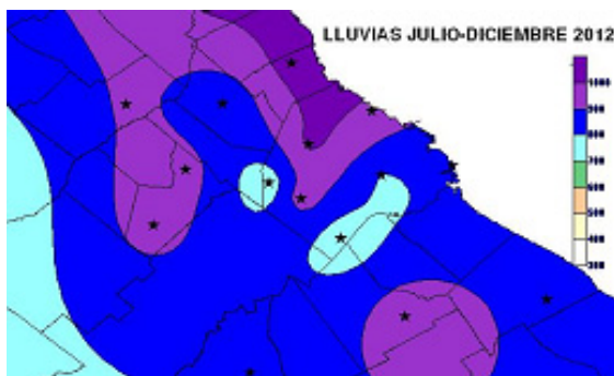
Figura 29: Lluvias (mm) julio a diciembre 2012
