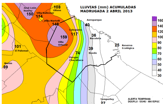
Figura 35: Lluvias 2 de abril de 2013 (madrugada)
