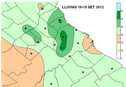
Figura 21: Lluvias (mm) 18-19 de septiembre de 2012
