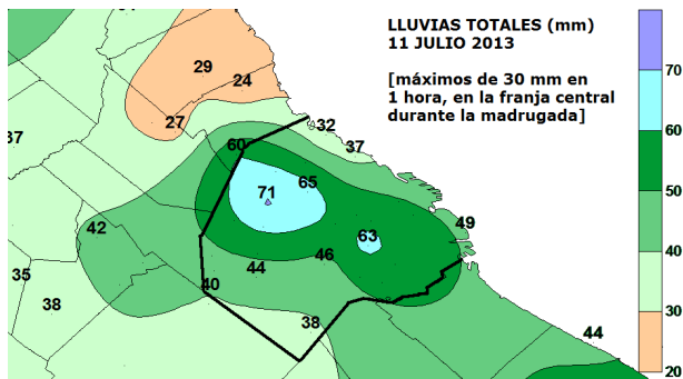
Figura 39: Lluvias 11 de julio de 2013
