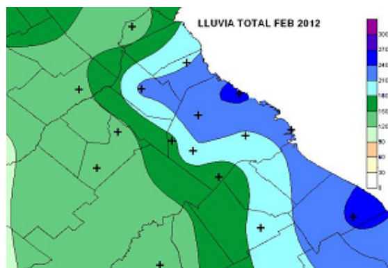
Figura 8: Lluvias totales (mm) febrero de 2012
