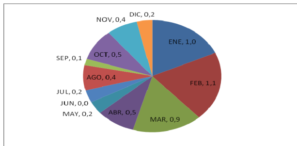
Figura 4: Frecuencia anual de días con más de 50 mm diarios (2001/10).
