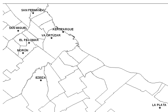
Figura 1: Estaciones meteorológicas del SMN
