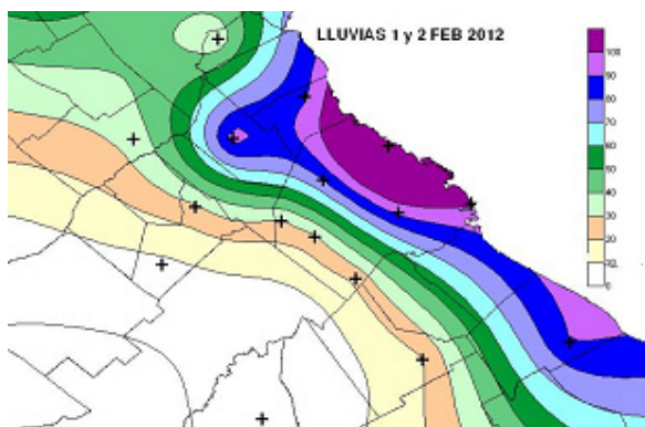
Figura 7: Lluvias (mm) 1 y 2 de febrero de 2012
