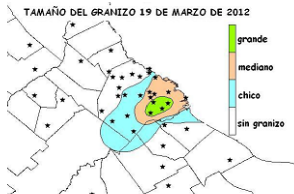
Figura 12: Tamaño del granizo del 19 de marzo
