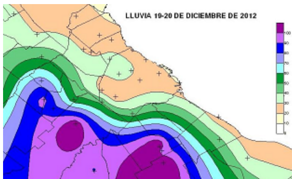
Figura 27: Lluvias (mm) 19-20 de diciembre de 2012
