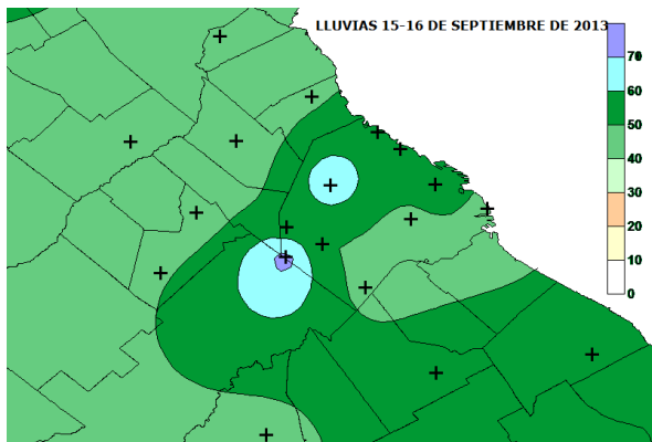
Figura 40: Lluvias del 15-17 de septiembre de 2013
