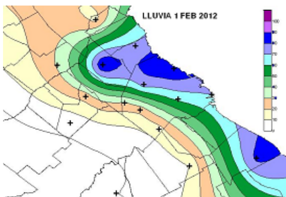
Figura 5: Lluvias (mm) 1° de febrero de 2012
