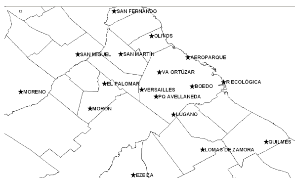
Figura 2: Estaciones SMN, GCBA y privados.
