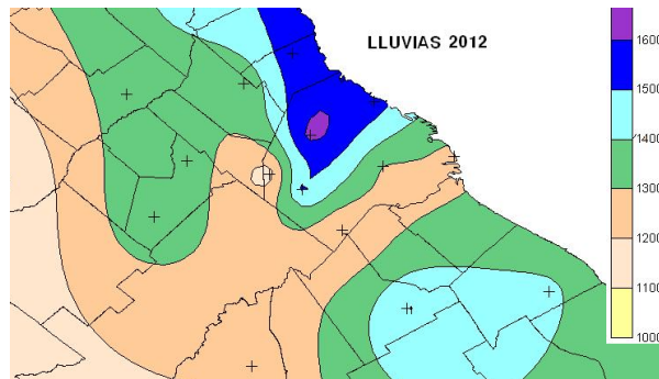
Figura 30: Lluvias totales (mm) en 2012.
