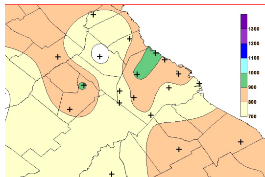
Figura 43: Lluvias totales del 2013 menos 1-2 de abril
