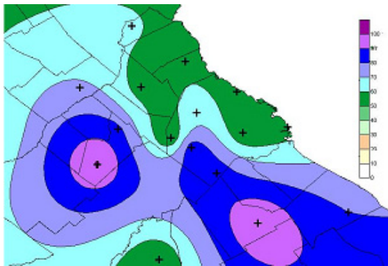
Figura 17: Lluvias (mm) 2-3 de agosto de 2012
