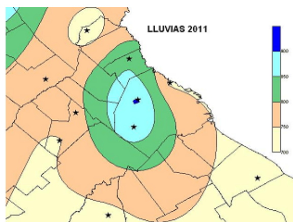
Figura 32: Lluvias totales (mm) en 2011.
