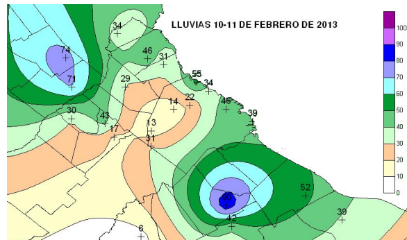
Figura 34: Lluvias (mm) 10-11 de febrero de 2013
