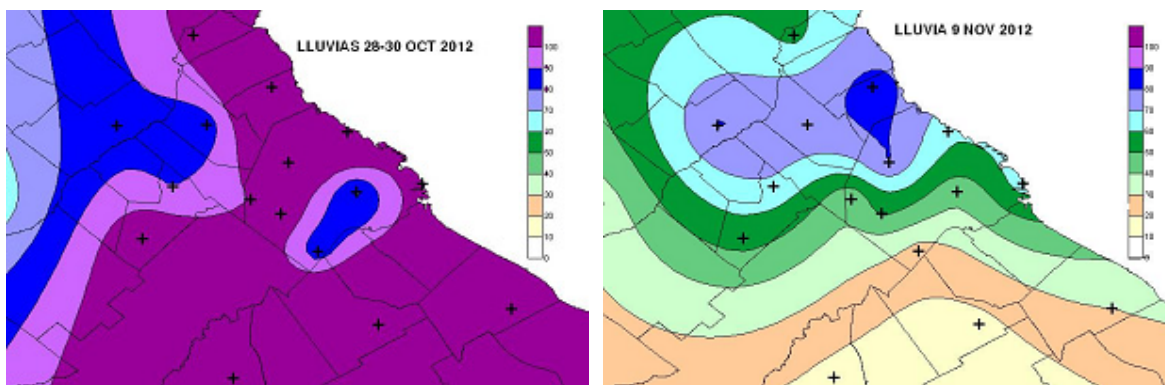
Figura 23: Lluvias (mm) 28 al 30 de octubre de 2012 Figura 24: Lluvias 9 de noviembre de 2012.
