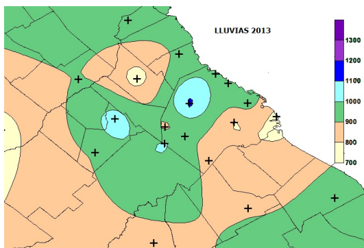
Figura 42: Lluvias totales (mm) del 2013
