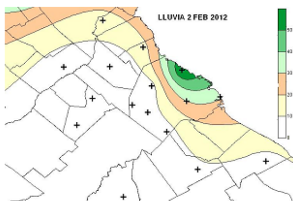
Figura 6: Lluvias (mm) 2 de febrero de 2012
