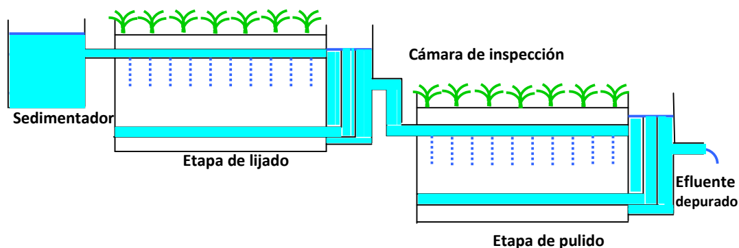
Figura 3.- Esquema de tratamiento por pantanos secos.
