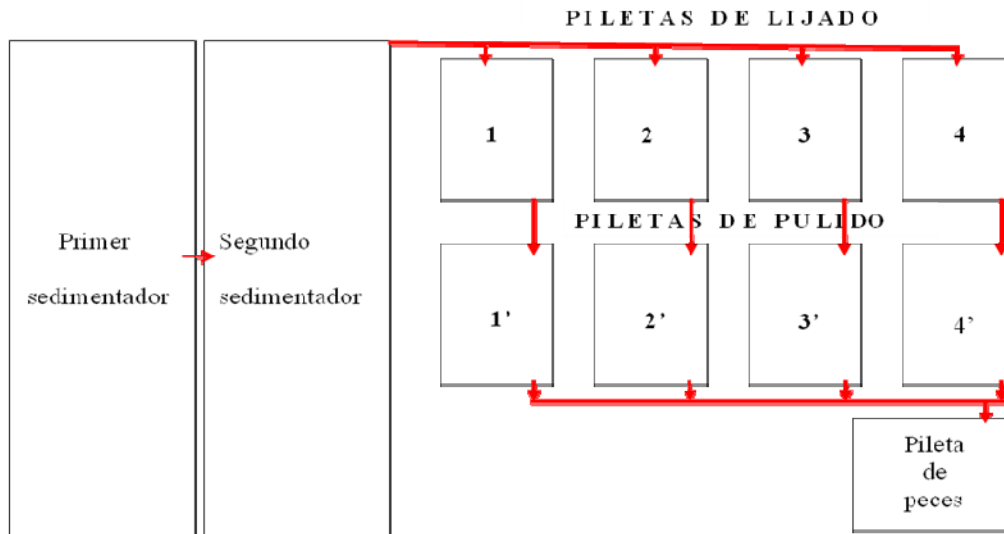
Figura 4.- Esquema de la instalación.
