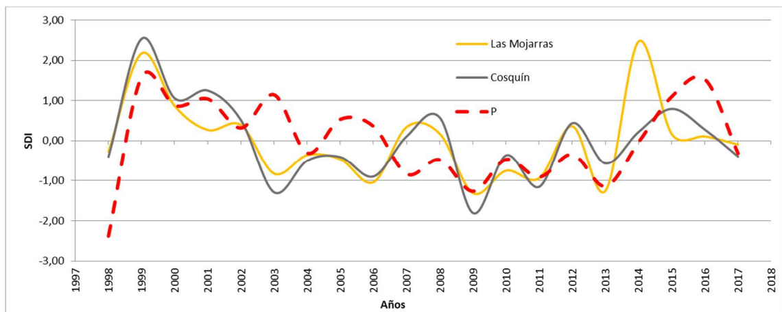
Figura 4.- Valores del índice SDI (k4) de la subcuenca del río Cosquín y del arroyo Las Mojarras. Además, se incorporan las precipitaciones representativas de la cuenca, normalizadas, a los fines comparativos. (1998-2017)
