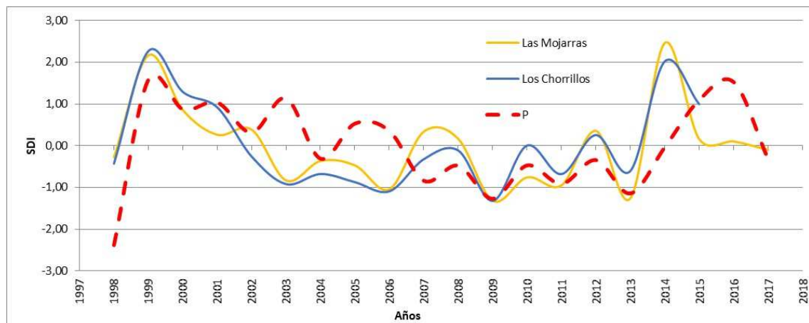
Figura 5.- Valores del índice SDI (k4) de la subcuenca del arroyo Las Mojarras y del arroyo Los Chorrillos. Además, se incorporan las precipitaciones representativas de la cuenca, normalizadas, a los fines comparativos. (1998-2017)
