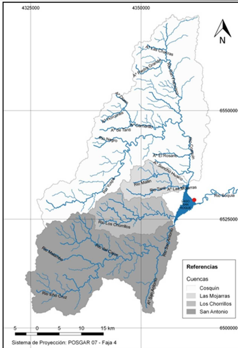
Figura 2.- Cuenca hidrográfica alta del río Suquia. Se destaca la estación pluviométrica Dique San Roque. (marca roja)
