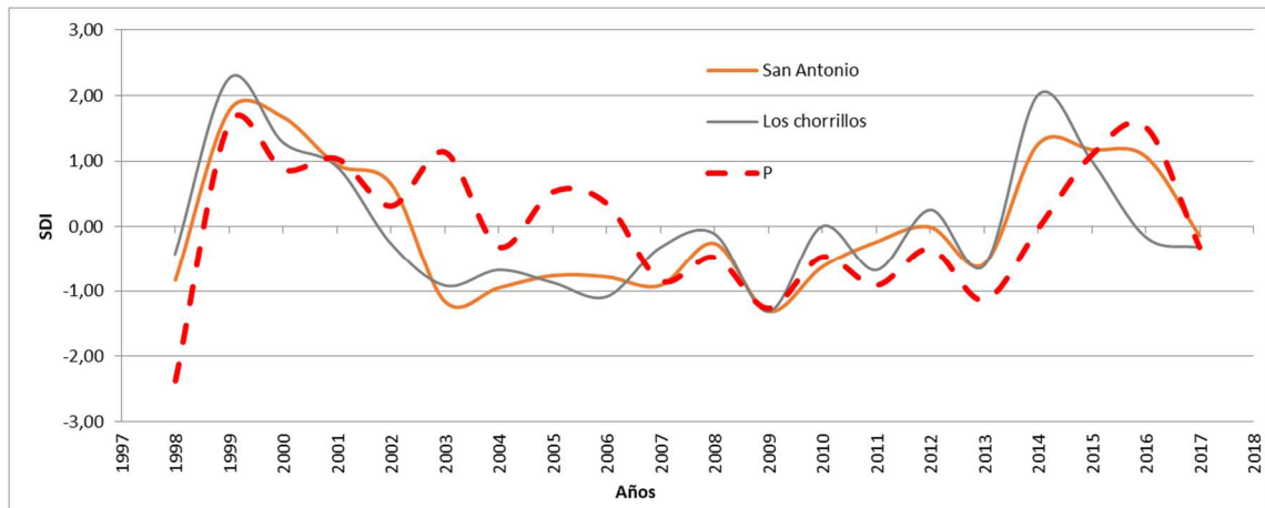
Figura 3.- Valores del índice SDI (k4) de la subcuenca del río San Antonio y del arroyo Los Chorrillos. Además, se incorporan las precipitaciones representativas de la cuenca, normalizadas, a los fines comparativos. (1998-2017)
