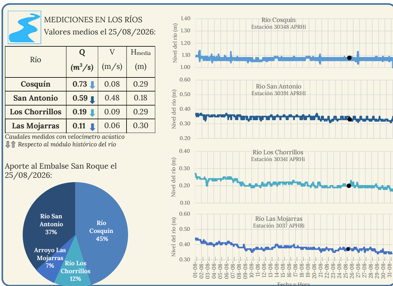
Figura 7. Resumen de las mediciones en los ríos el día 25/08/2026.
