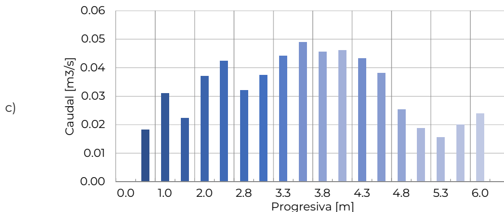
Figura 6. (a) Sección transversal del río San Antonio en el sitio de medición (b) perfil de velocidades medidos; (c) caudal aforado. La progresiva 0.00 corresponde con la margen derecha
