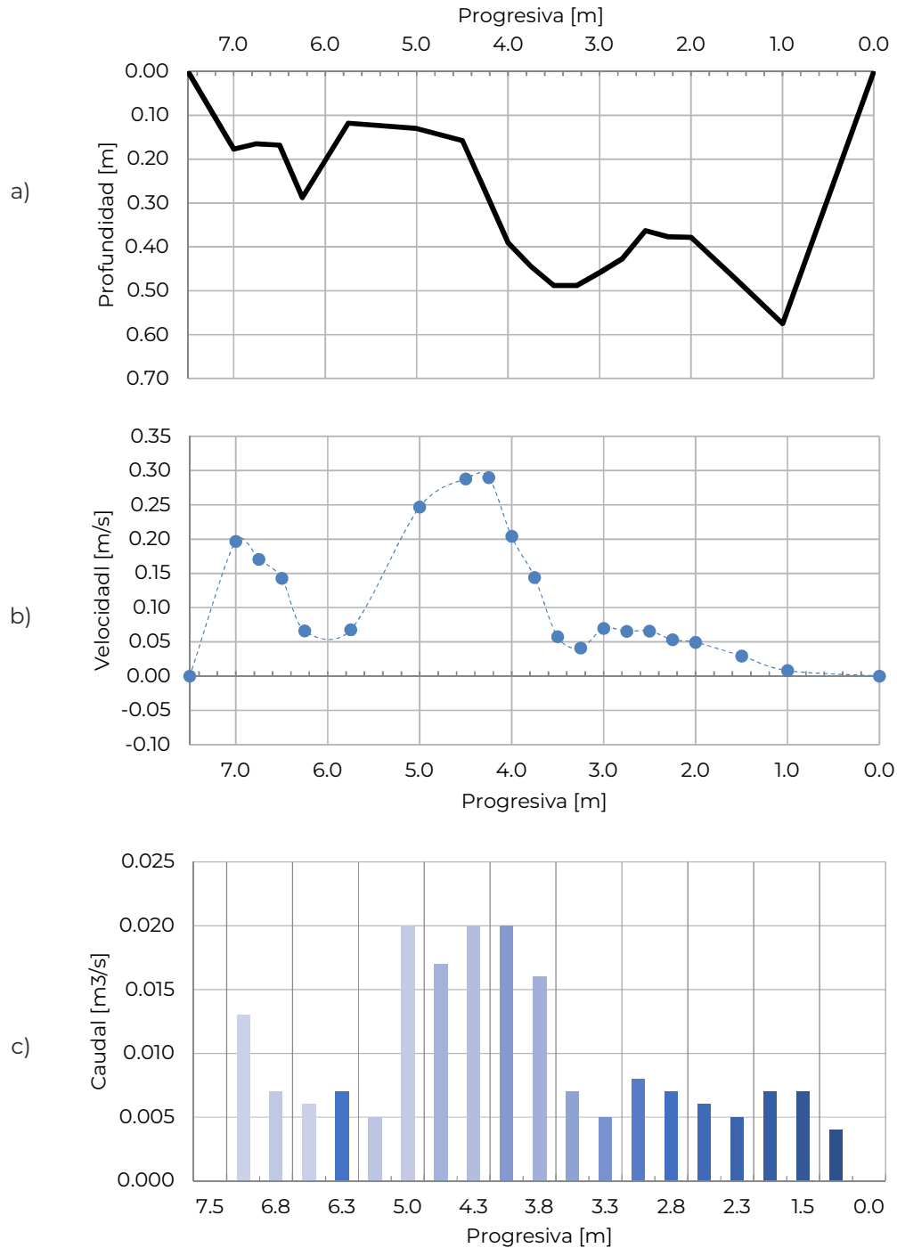
Figura 5. (a) Sección transversal del río Los Chorrillos en el sitio de medición, (b) perfil de velocidades medidos; (c) caudal aforado. La progresiva 0.00 corresponde con la margen derecha
