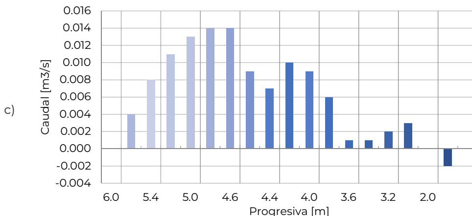
Figura 4. (a) Sección transversal del arroyo Las Mojarras en el sitio de medición (c) caudal aforado. La progresiva 0.00 corresponde con la margen izquierda
