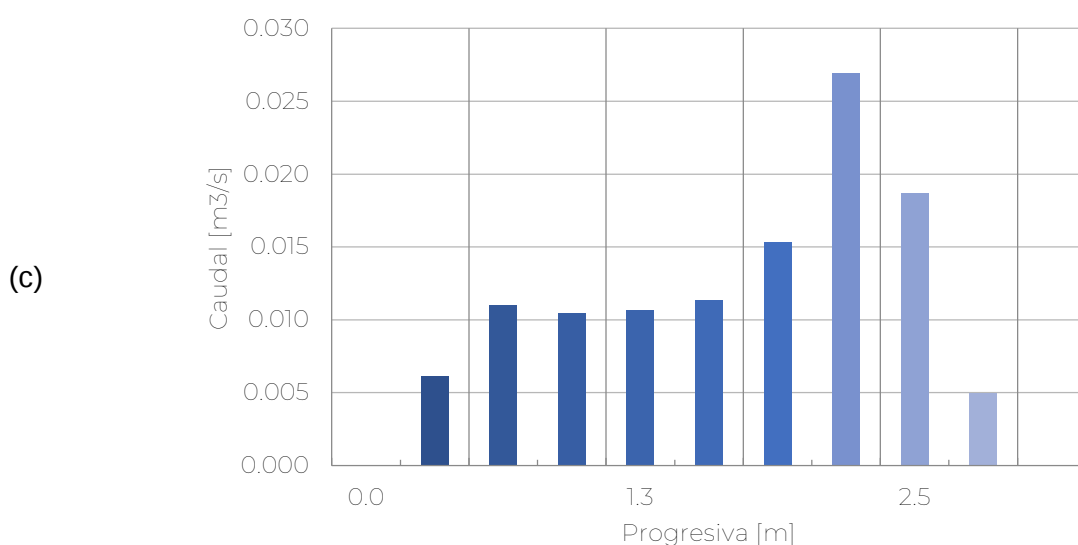
Figura 4.- (a) Sección transversal del arroyo Las Mojarras en el sitio de medición, (b) perfil de velocidades medido y (c) caudal aforado. La progresiva 0,00 se corresponde con la margen izquierda.
