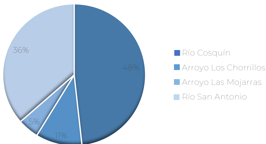
Figura 7. Caudales aportados por ríos tributarios al embalse San Roque, el día 24/06/2025.
