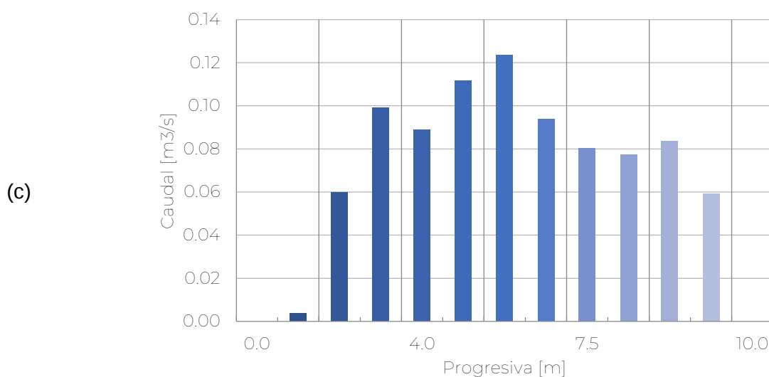
Figura 6.- (a) Sección transversal del río San Antonio en el sitio de medición, (b) perfil de velocidades medido y (c) caudal aforado. La progresiva 0.00 se corresponde con la margen izquierda.
