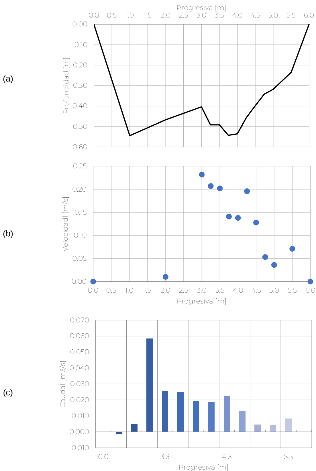
Figura 5.- (a) Sección transversal del arroyo Los Chorrillos en el sitio de medición, (b) perfil de velocidades medido y (c) caudal aforado. La progresiva 0,00 se corresponde con la margen izquierda.
