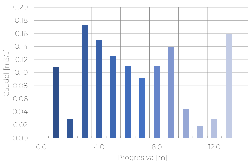
Figura 6.- (a) Sección transversal del río San Antonio en el sitio de medición, (b) perfil de velocidades medido y (c) caudal aforado. La progresiva 0.00 se corresponde con la margen izquierda.
