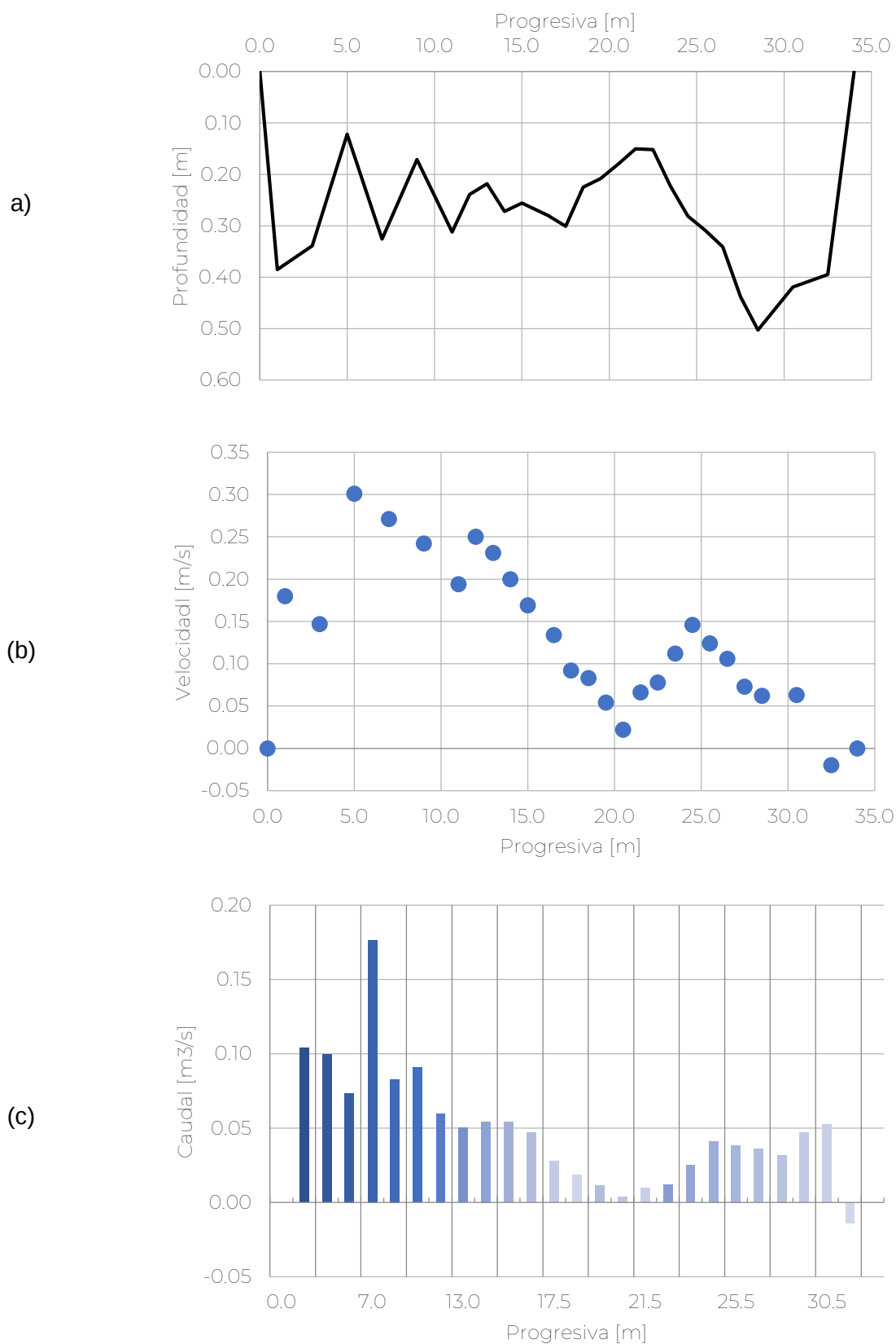
Figura 3.- (a) Sección transversal del río Cosquín en el sitio de medición, (b) perfil de velocidades medido y (c) caudal aforado. La progresiva 0,00 se corresponde con la margen izquierda.
