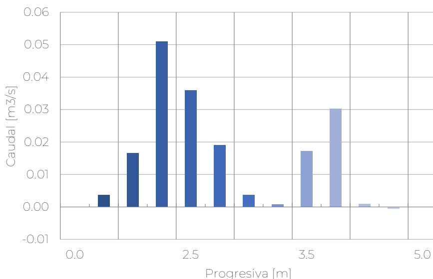
Figura 4.- (a) Sección transversal del arroyo Las Mojaras en el sitio de medición, (b) perfil de velocidades medido y (c) caudal aforado. La progresiva 0,00 se corresponde con la margen izquierda.
