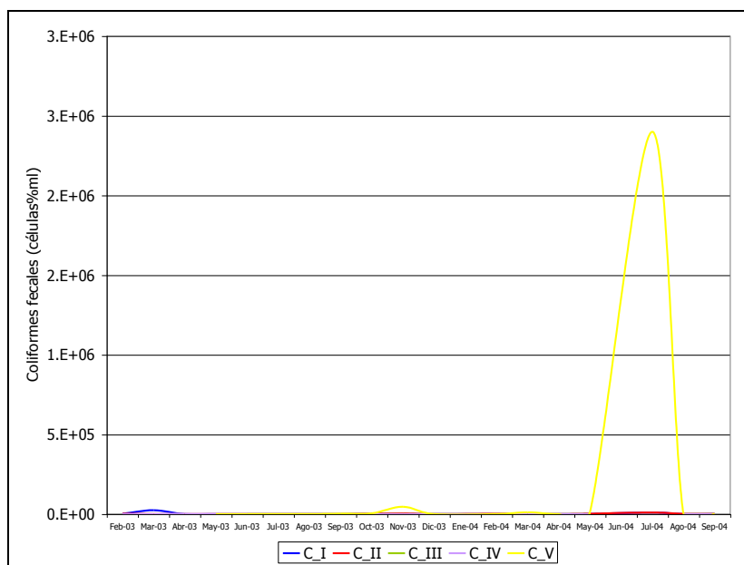
Figura 25: Variación temporal de fecales en canales
