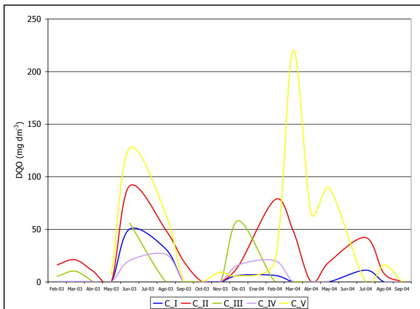
Figura 15: Variación temporal de DQO en canales
