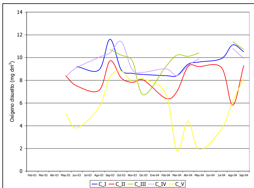
Figura 16: Variación temporal de OD en canales
