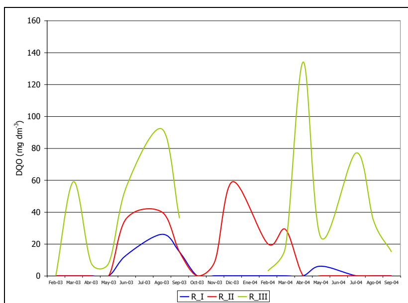
Figura 13: Variación temporal de DQO en el río
