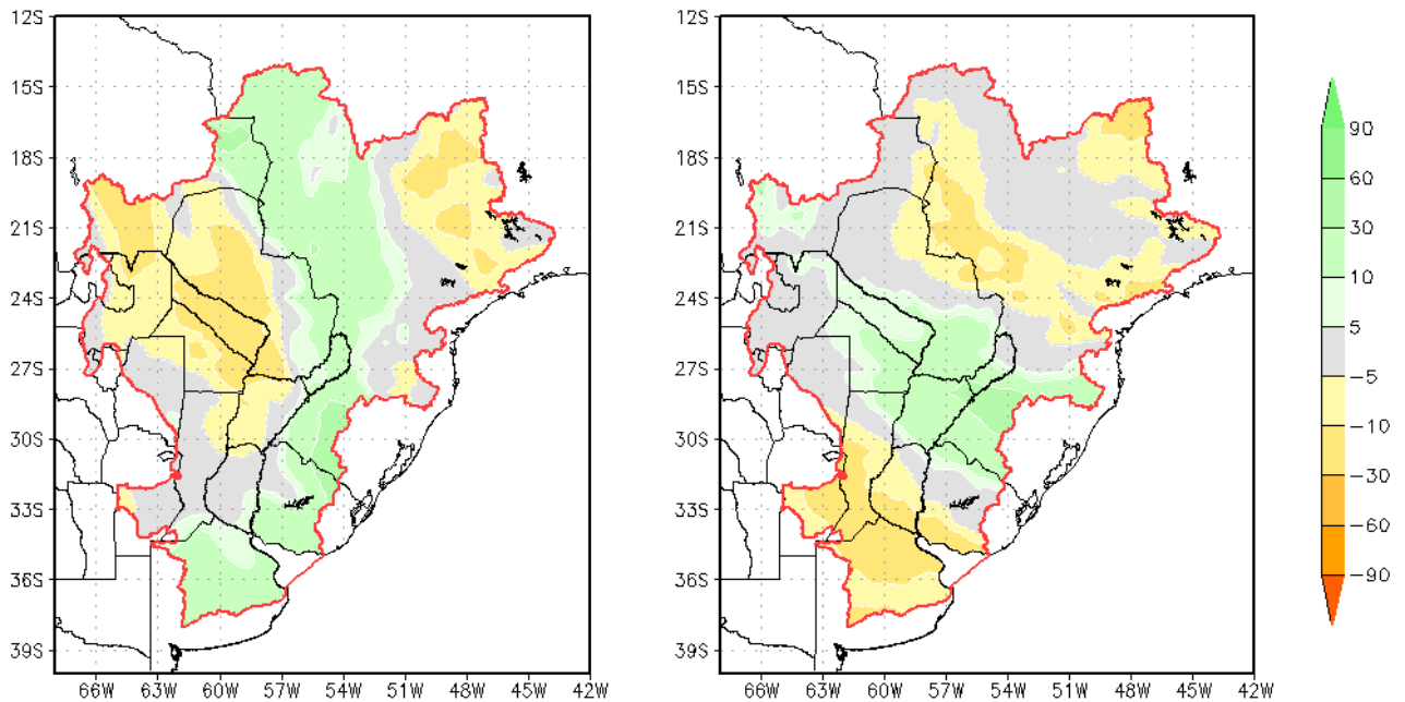
Figura 5: Pronóstico numérico de la anomalía de la precipitación acumulada semanal (mm, somb.) respecto a la climatología del modelo EGFS (2000-2019) para la semana 1 (15/04 al 22/04 12 UTC) y la semana 2 (23/04 al 29/04 12 UTC) .
